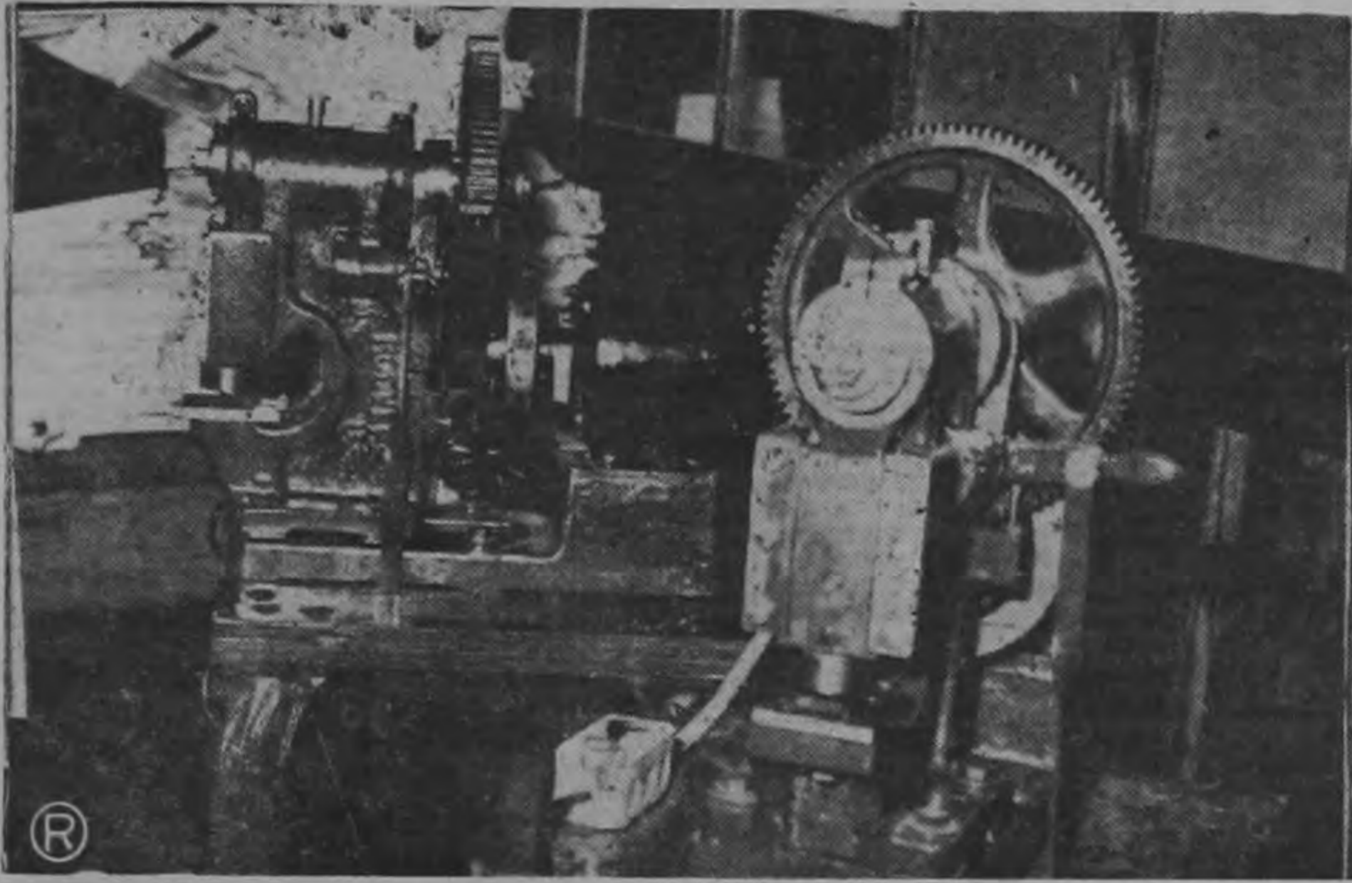
MAQUINAS SELLADORAS DANADAS: — Estas son las máquinas selladoras automáticas pedidas por el Tribunal Supremo de Elecciones para el servicio del Registro Civil, cuyos sellos o troqueles se extraviaron al romperse las cajas de madera en que venían. Nótese en la rueda dentada arriba, que no tiene el cobertor correspondiente, y también faltan otras piezas que ya fueron pedidas. Los sellos de estas máquinas fueron pedidos nuevamente a los Estados Unidos, pero son diferentes a los extraviados. (FOTO SOLANO)
